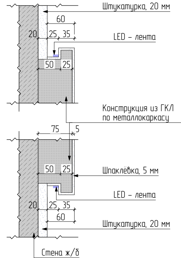
Д1 (Конструкция за ТВ)
