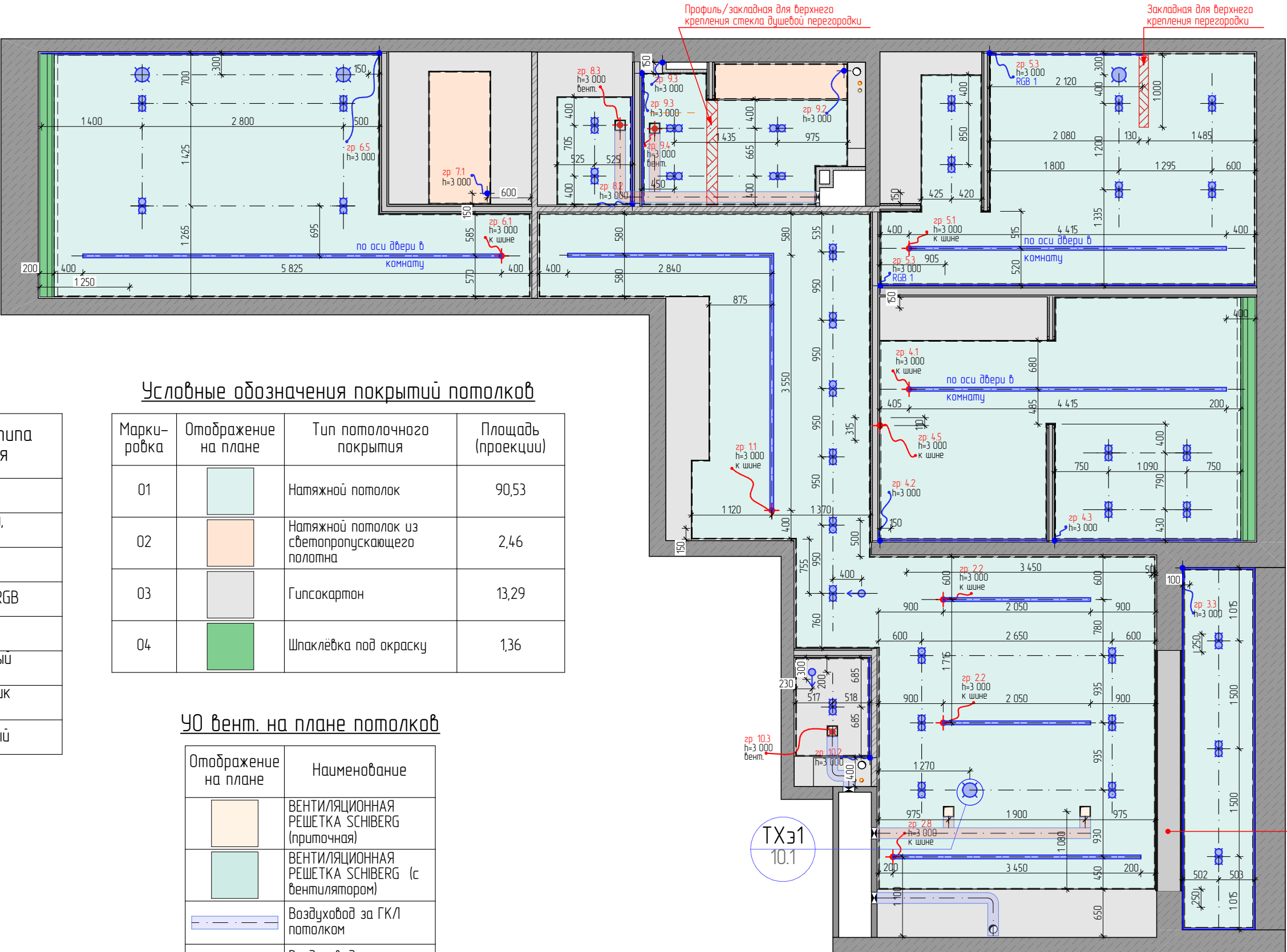
УО на плане потолков
