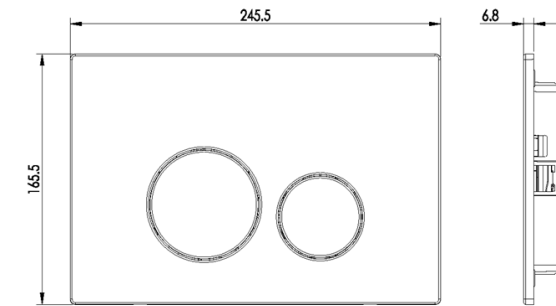
TX9 Клавиша смыва (туалет)
