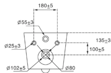
TX10 Унитаз (туалет)
