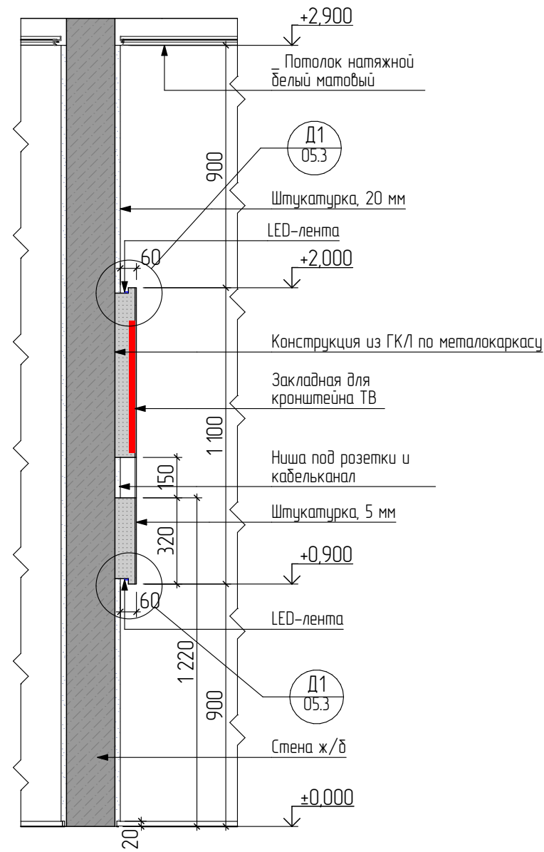
Сечение 1-1 (Конструкция за ТВ)
