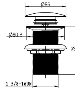
TX8 Донный клапан
