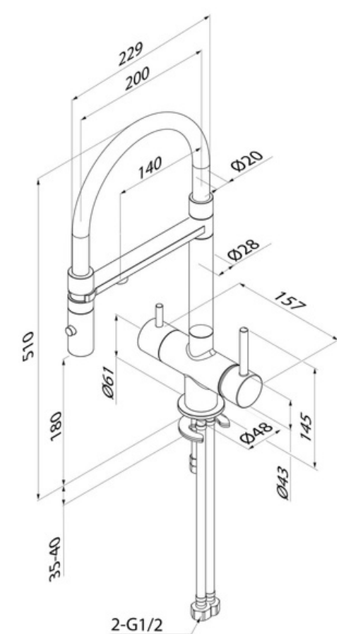
TX3 Смеситель для кухни
