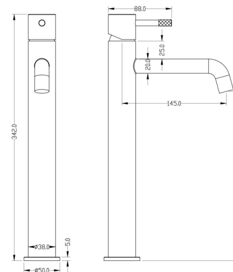
TX11 Смеситель для раковины (туалет)
