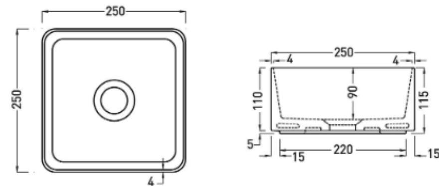
TX12 Раковина (туалет)
